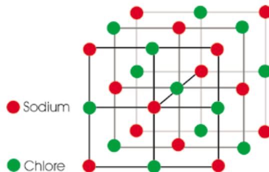
Schéma d'un cristal cubique de chlorure de sodium.
